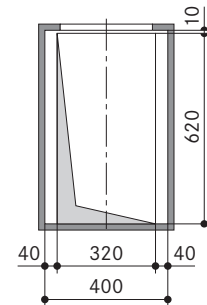
Übergabebereich 2 (Maße ohne Drehvorrichtung)
