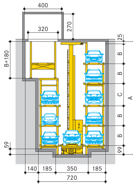
Übergabebereich 2 (Maße ohne Drehvorrichtung)
